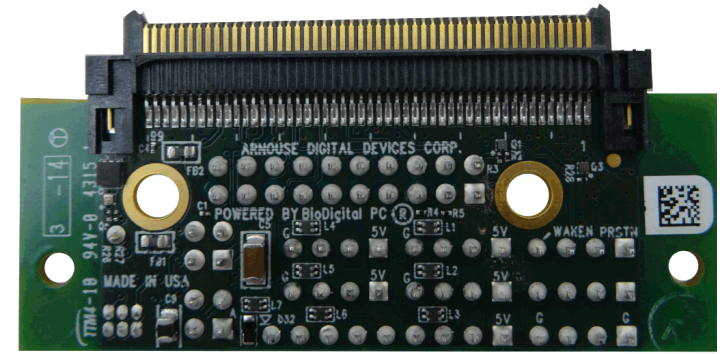
PCB BOTTOM
